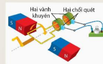
Hình 14.9 Minh họa cách tạo ra dòng điện xoay chiều
