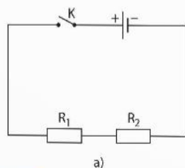
Hình 12.1 Sơ đồ đoạn mạch nối tiếp (a) và mạch điện có hai bóng đèn mắc nối tiếp (b)
