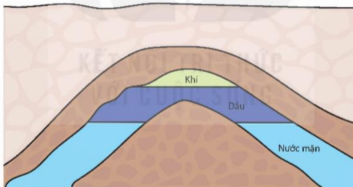
Hình 25.1 Sơ đồ cấu tạo mỏ dầu
