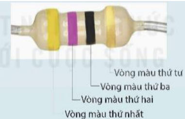
Hình 11.4 Điện trở bốn vòng màu
