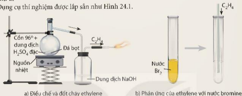
Hình 24.1 Điều chế ethylene và thử tính chất
