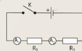
Hình 12.2 Sơ đồ mạch điện của thí nghiệm tìm hiểu đặc điểm mạch nối tiếp
