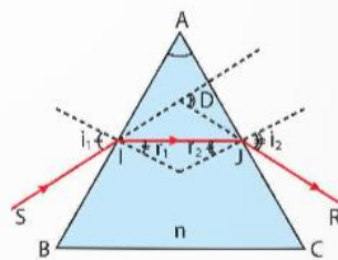
Hình 7.6 Đường truyền của tia sáng qua lăng kính
