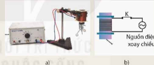
Hình 15.4 Thí nghiệm về tác dụng từ của dòng điện xoay chiều (a) và sơ đồ mô tả thí nghiệm (b)
