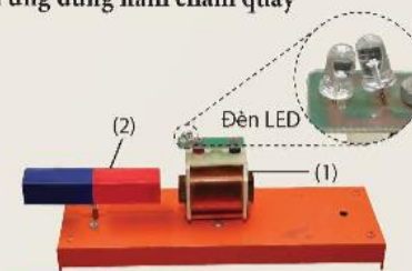
Hình 14.4 Thí nghiệm dùng nam châm quay
