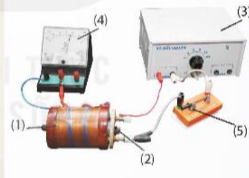
Hình 14.3 Thí nghiệm về dòng điện cảm ứng dùng nam châm điện
