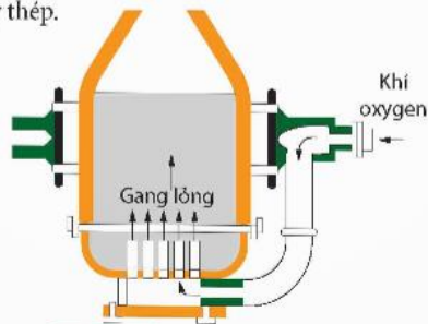
Hình 20.3 Sơ đồ lò thổi
