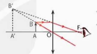
Hình 10.4 Sơ đồ tạo ảnh qua kính lúp khi d < f
