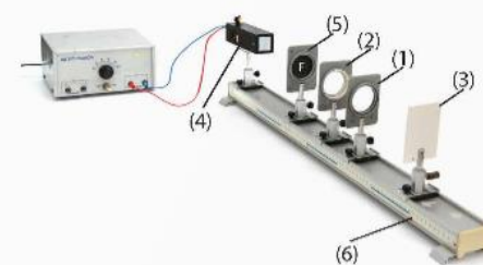
Hình 1.3 Bộ dụng cụ tìm hiểu tính chất ảnh qua thấu kính
