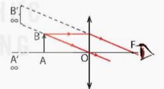
Hình 10.5 Sơ đồ tạo ảnh qua kính lúp khi d = f
