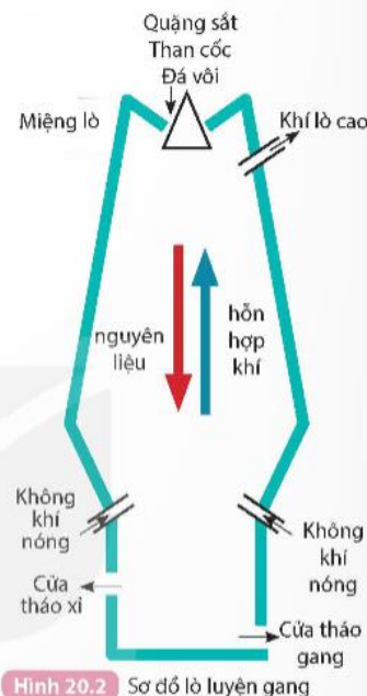
Hình 20.2 Sơ đồ lò luyện gang
