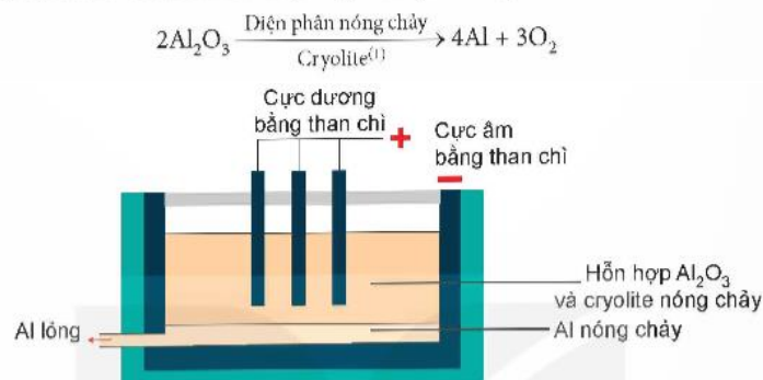
Hình 20.1 Sơ đồ bể điện phân aluminium oxide nóng chảy
