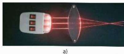
Hình 8.3 Đường truyền của ba chùm sáng hẹp, song song qua thấu kính hội tụ (a) và qua thấu kính phân kì (b)
