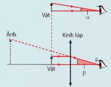
Hình 10.3 Góc trông vật (a) và góc trông ảnh của vật qua kính lúp (b)
