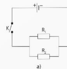
Hình 12.3 Sơ đồ đoạn mạch song song (a) và mạch điện có hai bóng đèn mắc song song (b)
